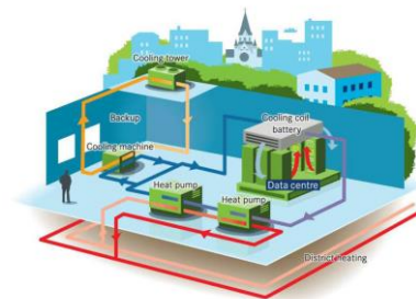
Géothermie (Stockholm)
